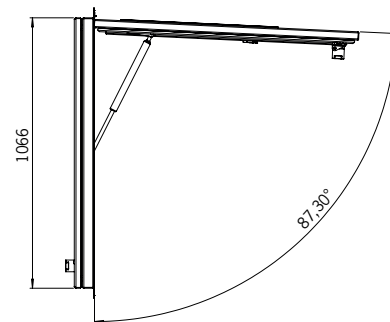
Panoramaklappe geöffnet - Seitenansicht -
